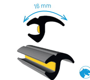
Profil universel « tenue extrême » Profil PB 16 mm avec butyl rouleau 22,8 m M16L • REF : PP-JT022
