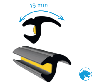
Profil universel « tenue extrême » Profil PB 19 mm avec butyl rouleau 22,8 m M19L • REF : PP-JT023
