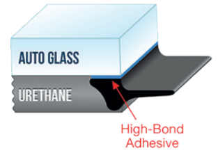
Profil intérieur PB PUGM4 • 6 mm x 23 m REF : PP-JT122
