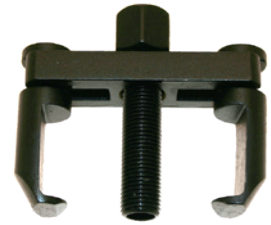
Arrache essuie-glace (bras réglables) Le trou dans l'axe permet de déposer les bras d'essuie-glace avec gicleur incorporé REF : PP-WST51F
