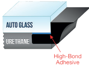
Profil intérieur PB PUGM2 • 7 mm x 23 m REF : PP-JT121
