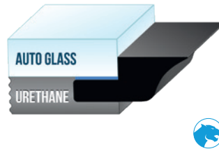
Profil intérieur PB « mousse » PUGM3 • 8 mm x 23 m avec adhésif REF : PP-JT099
