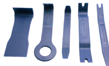
Jeu de 5 outils plastique pour déposer la garniture REF : PP-GT0006
